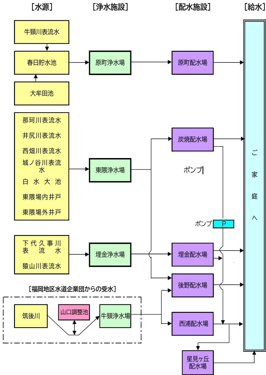
図-2 水源からご家庭までの給水フロー図
